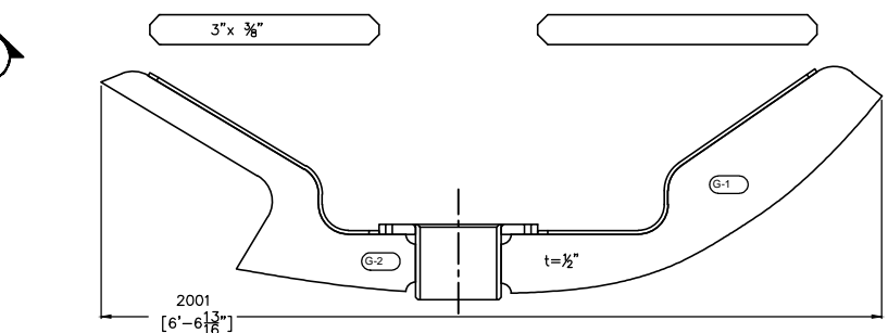
SECTION G SCALE: 1:10
