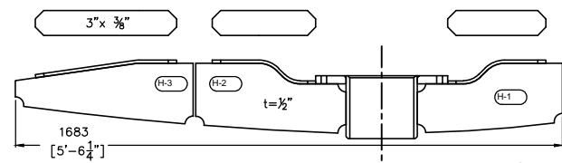
SECTION H SCALE: 1:10
