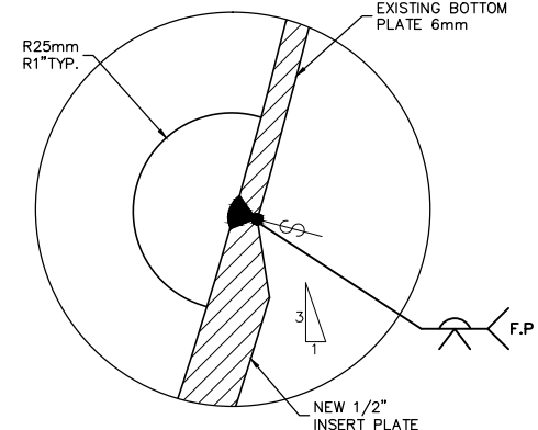
DETAIL K SCALE: 1:1
