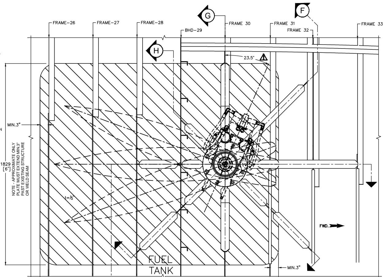
SECTION E SCALE: 1:10
