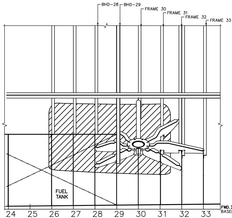
SECTION C SCALE: 1:20
