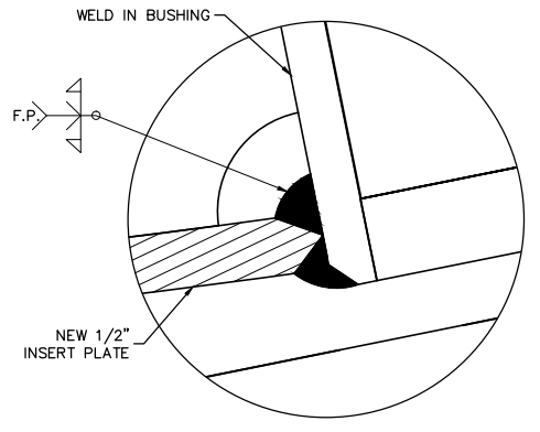
DETAIL L SCALE: 1:1
