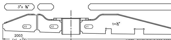
SECTION J SCALE: 1:10
