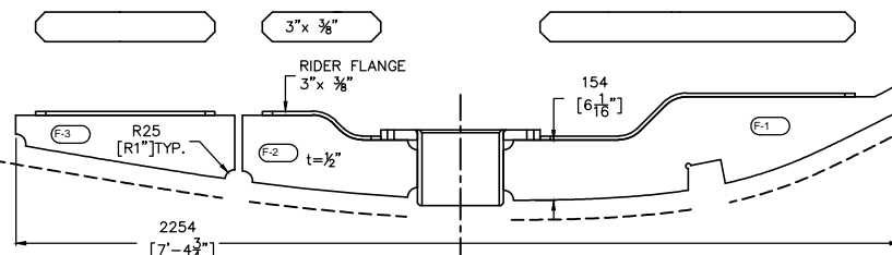
SECTION F SCALE: 1:10
